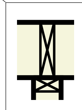
Схема Т-образного соединения стен
