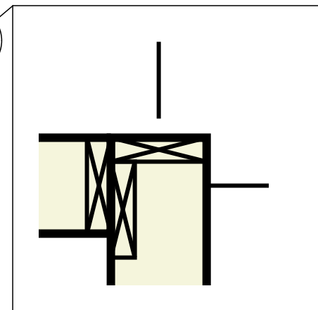
Схема углового соединения стен
