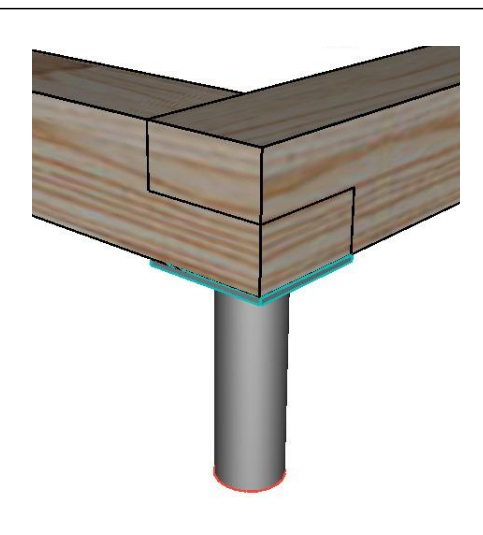
Узел Б
