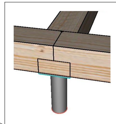
Узел Б
